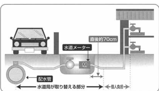
専用水道・簡易水道などの鉛製給水管
