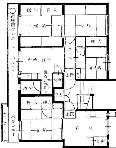
ペア住宅(第二種)間取り
