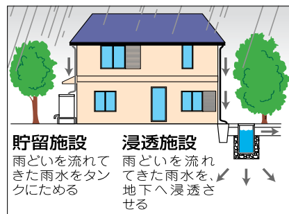
貯留施設 雨どいを流れてきた雨水をタンクにためる
